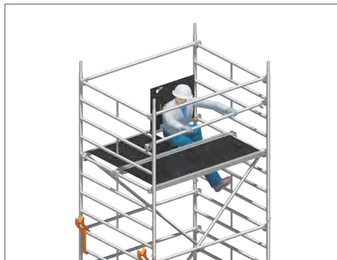
4. Montage der Zwischengeländer aus gesicherter Position im Bereich der Durchstiegsklappe.
