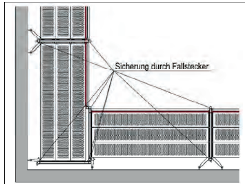
Bild 2-41: Gerüst an innen liegender Ecke (Beispiel)
