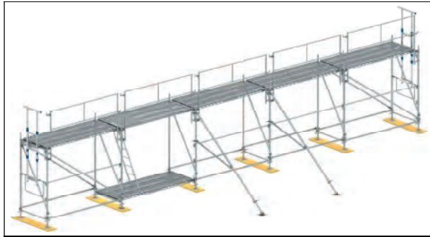
Bild 2-35: Vorübergehende Kippsicherung der 1. Gerüstlage mit Gerüststützen
