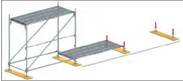
Bild 2-3: Fertiggestelltes erstes Gerüstfeld eines Gerüsts der Lastklasse \leq 4 , Ausführung bei geplantem Weiterbau mit Montage-Sicherungs-Geländer
