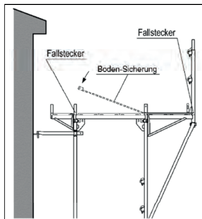
Bild 2-1: Beispiel: Boden-Sicherung bei Konsolkonfiguration 2 mit Geländerstütze
