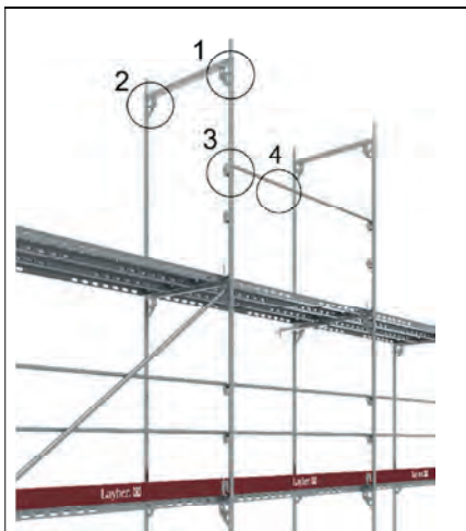
Bild 2-10: Anschlagpunkte 1, 2, 3 und 4 für PSAgA (Details siehe Bilder 2-11, 2-12 und 2-13)
