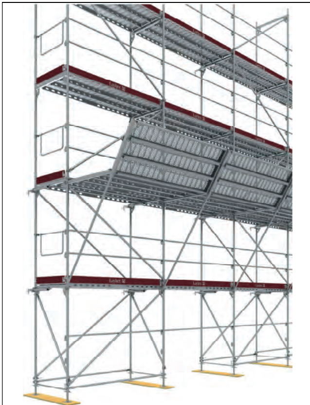
Bild 3-5: Grundkonfiguration mit Schutzdach
