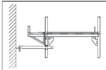
Bild 2-43: „Gerüsthalter kurz“
