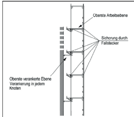
Bild 2-39: Oberste Arbeitsebene unverankert, Beispiel für Feldlänge \leq 2,07\text{ m}
