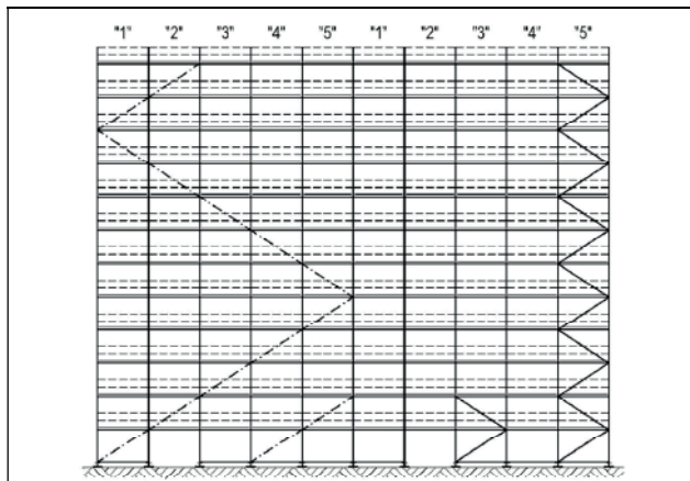
Bild 2-2: Anordnung der Vertikaldiagonalen und Horizontalstreben, Mindestausstattung. Informationen zur Anordnung der Vertikaldiagonalen und Horizontalstreben innen/außen: siehe Systemkonfigurationen der Regelausführung.
