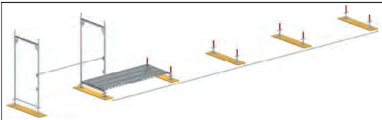
Bild 2-22: Vorbereitung des Aussteifungsfeldes
