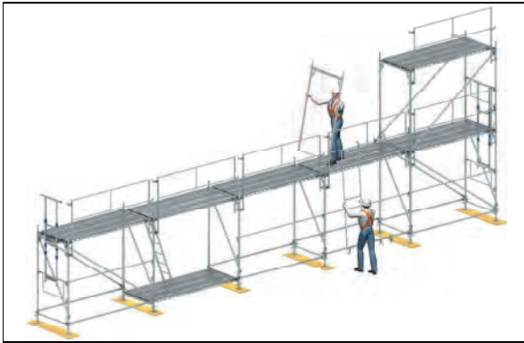
Bild 2-31: Montage der Gerüstfelder (I)
