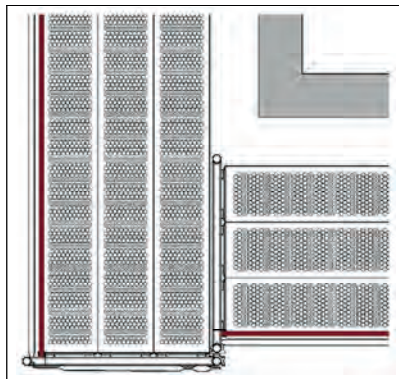
Bild 2-38: Eckausbildung (Draufsicht)
