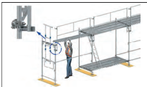
Bild 2-9: Durch Kupplung gesichertes linkes Ende einer I-Geländerkette
