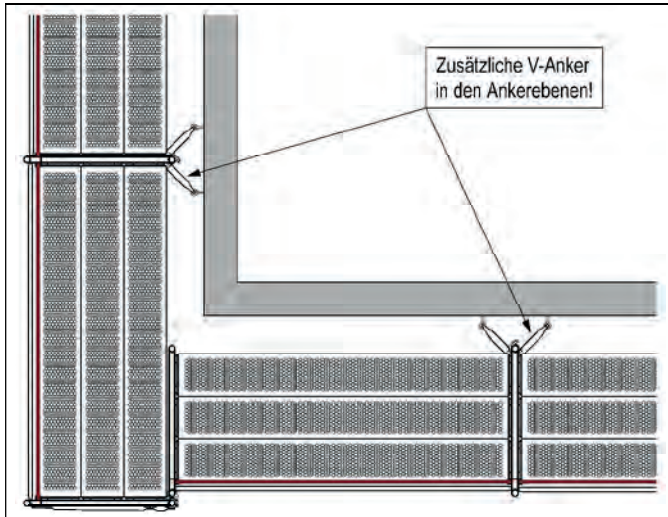
Bild 2-46: Zusätzliche V-Anker an einer Außenecke
