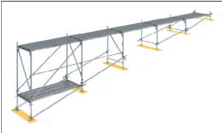
Bild 2-20: Geländeausgleich; Ausführungsbeispiel für den Weiterbau mit Montage-Sicherungs-Geländer
