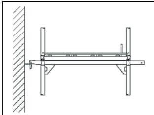
Bild 2-42: „Gerüsthalter lang“
