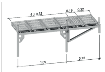
Bild 3-10: Anordnung der Böden bei Außenkonsole 0,73 m
