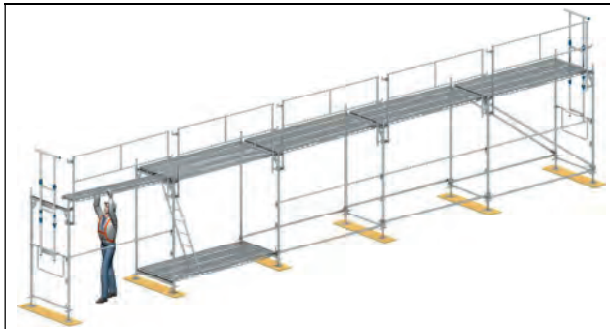
Bild 2-30: Montage des letzten Gerüstfeldes der untersten Lage, mit Stirn-Montage-Sicherungs-Geländer (Diagonalen, Horizontalstreben und Querdiagonale im letzten Feld sind noch nicht eingebaut)
