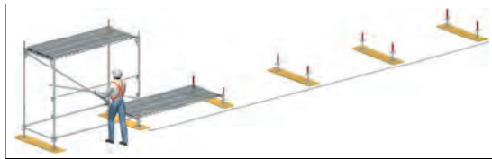
Bild 2-23: Fertigstellung des Aussteifungsfeldes
