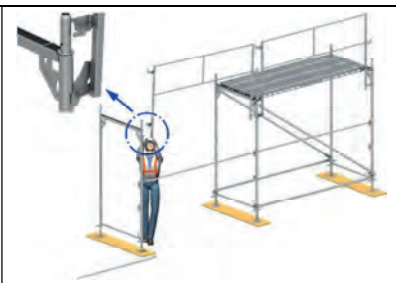
Bild 2-8: Montage I-Geländer (2)
