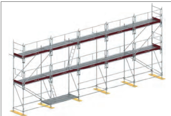
Bild 2-33: Fertig montiertes Gerüst
