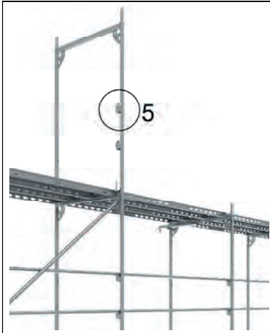
Bild 2-14: Anschlagpunkt 5 für PSaGA (Detail siehe Bild 2-16)
