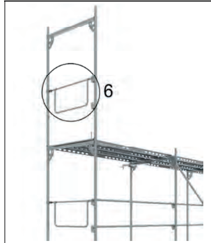
Bild 2-15: Anschlagpunkte 6 für PSaGA (Details siehe Bilder 2-17a, 2-17b)
