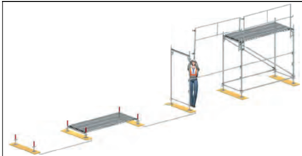
Bild 2-29: Montage des I-Geländers im zweiten Gerüstfeld
