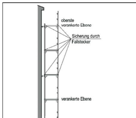
Bild 2-40: Gerüst an Gebäude mit geringer Dachneigung
