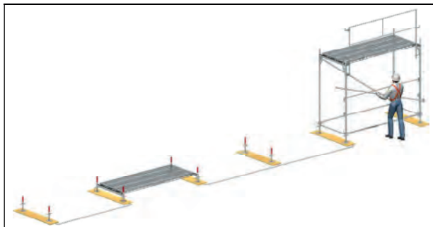
Bild 2-28: Montage des Aussteifungsfeldes mit I-Geländer
