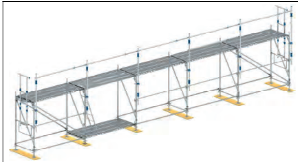
Bild 2-25: Vorübergehende Sicherung der aktuell obersten Lage mit dem Montage-Sicherungs-Geländer
