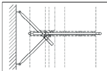
Bild 2-45: V-förmig angeordnetes Ankerpaar
