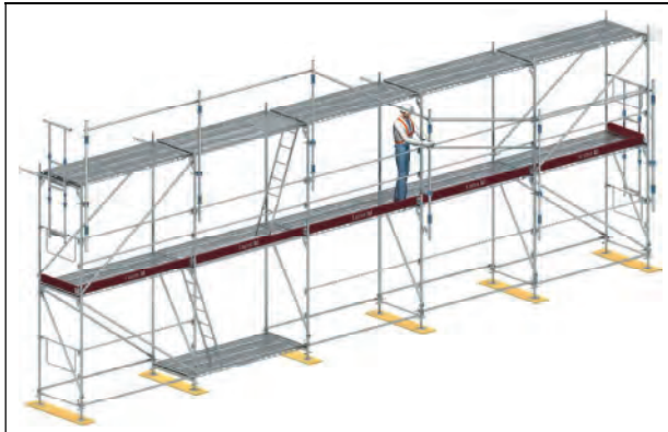
Bild 2-27: Umsetzen des Montage-Sicherungs-Geländers von der gesicherten Lage aus
