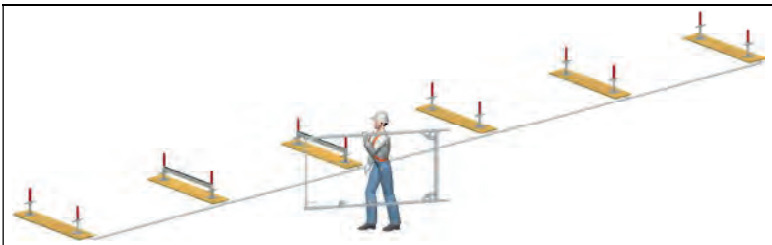
Bild 2-21: Auslegen der untersten Gerüstlage
