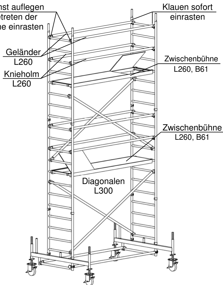
Bild 10: Zwischenbühne Standhöhe 4.40 m
