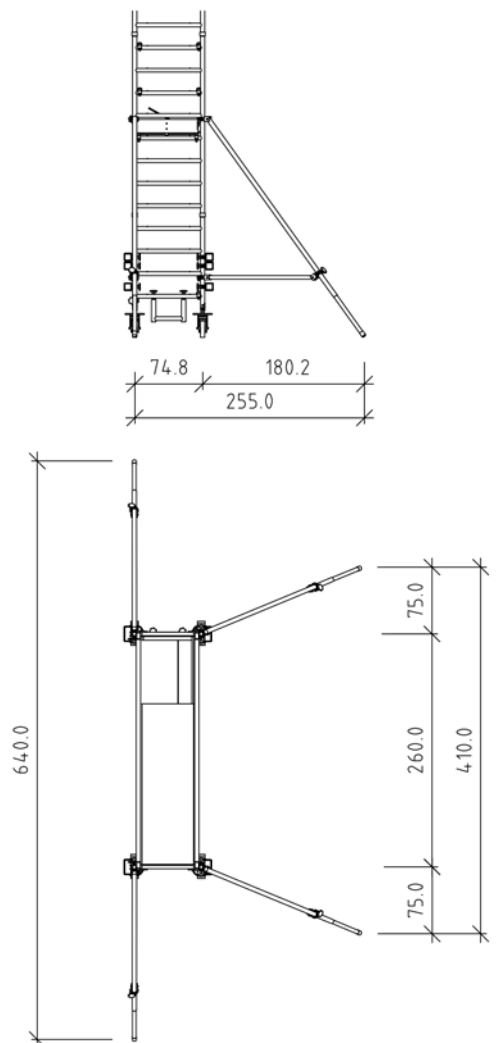
Bild 17: wandseitiger Aufbau
