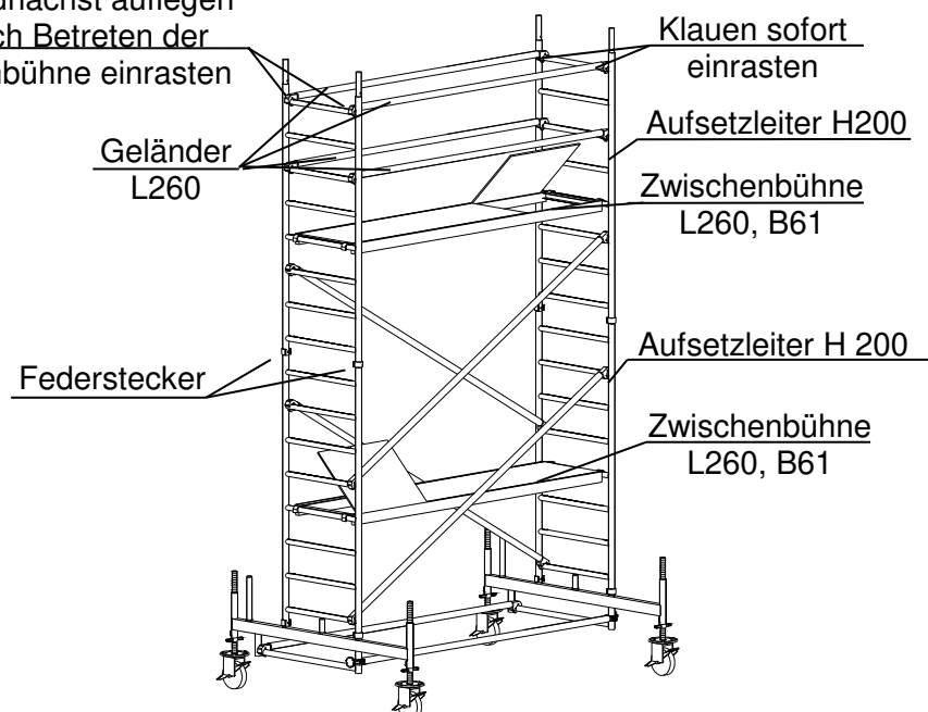
Bild 11: Zwischenbühne Standhöhe 3.40 m
