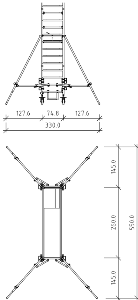
Bild 16: mittiger Aufbau
