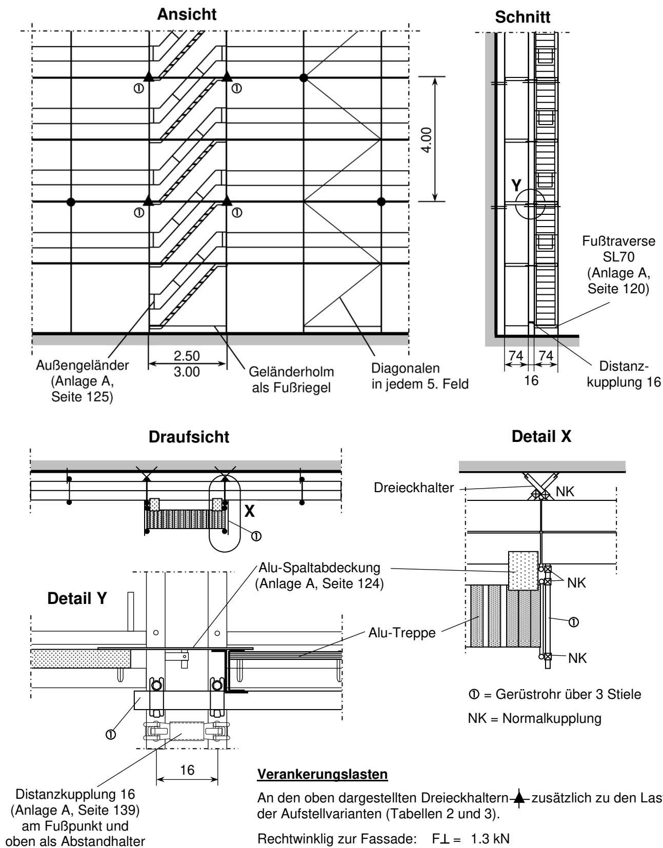
Bild 60: Gleichläufiger Treppenaufstieg
