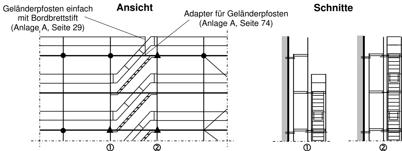
Bild 62: Oberer Abschluss gleichläufige Treppe
