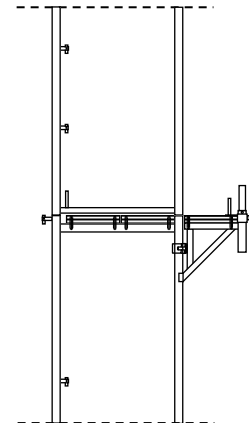
Bild 23: Konsole 32
