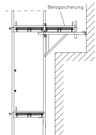
Bild 24: Konsole 64
