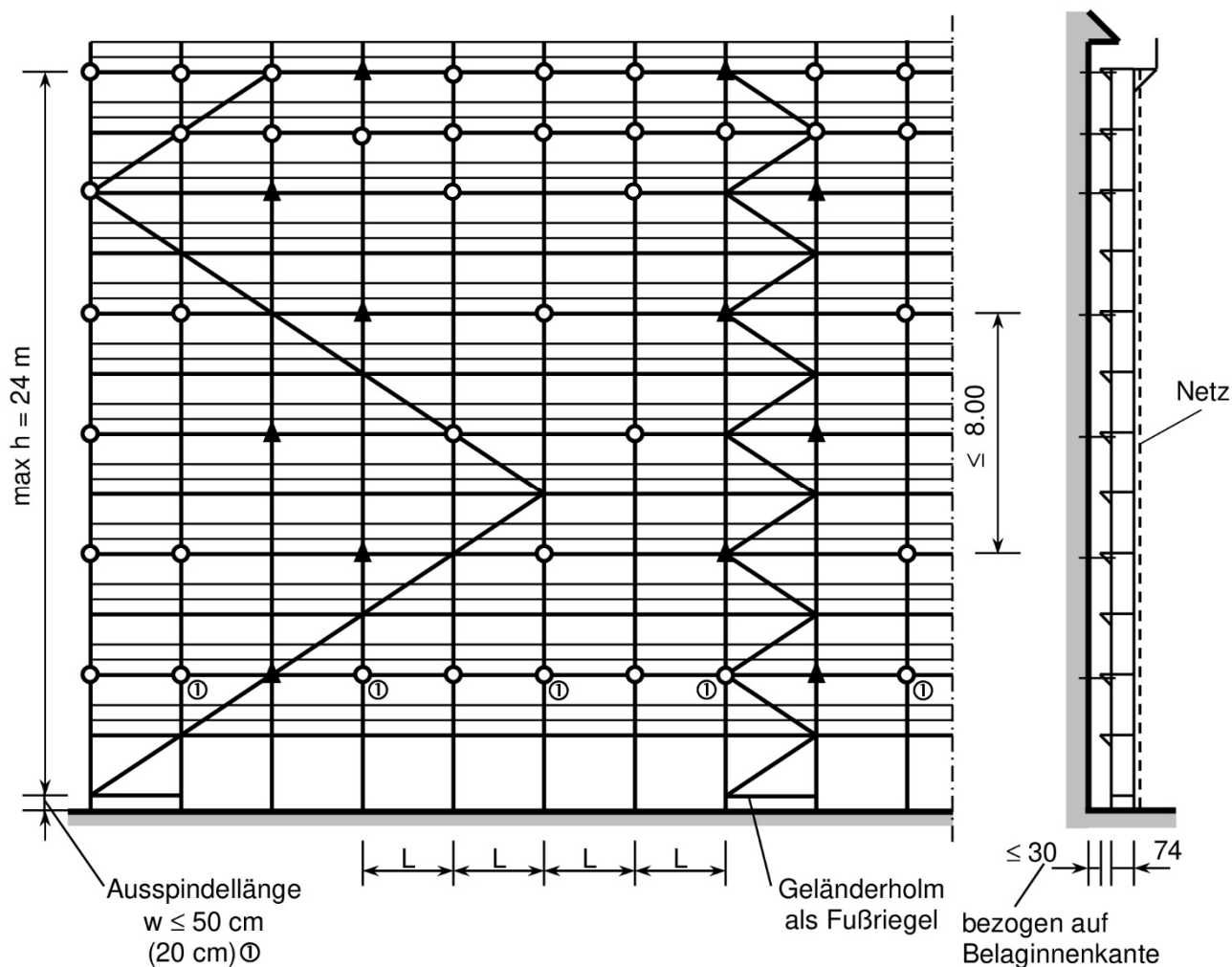
Bild 34: Konsolvariante 2 (Konsole 74 ohne lange Strebe), L = 3.00 m ohne Schutzwand in der obersten Ebene, Ankerraster: 8 m versetzt mit Netzbekleidung vor geschlossener Fassade
