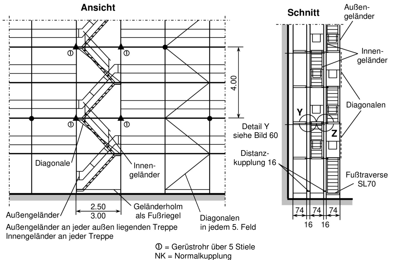
Bild 61: Gegenläufiger Treppenaufstieg
