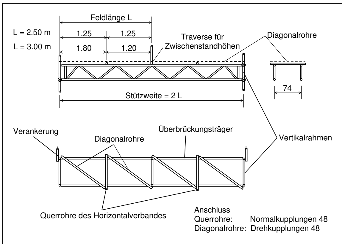
Bild 54: Aussteifung der Überbrückungsträger mit Horizontalverband
