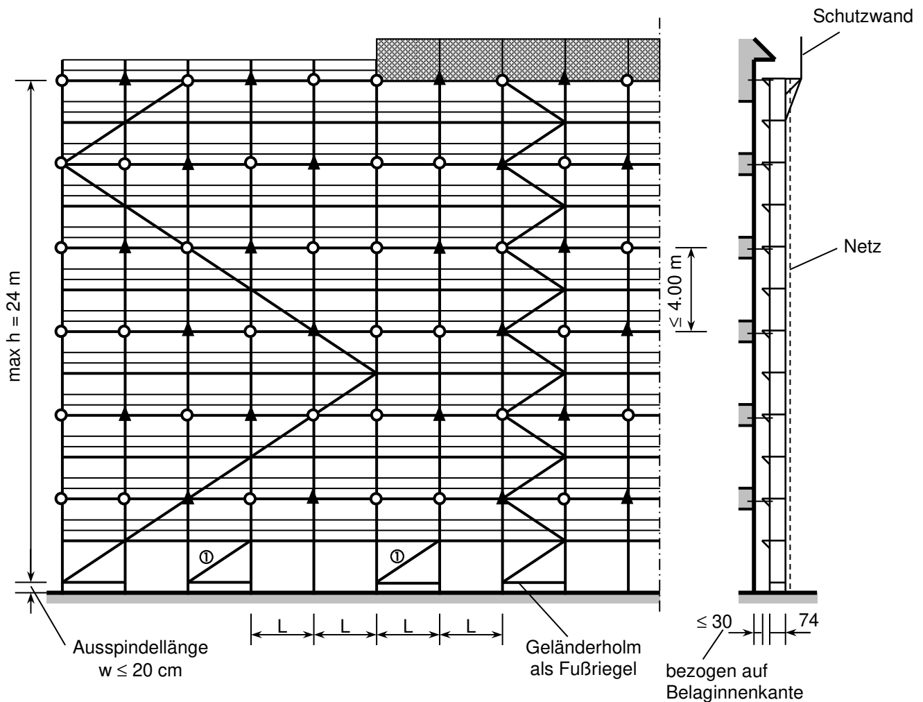
Bild 41: Gerüst mit Netzbekleidung vor teilweise offener Fassade
