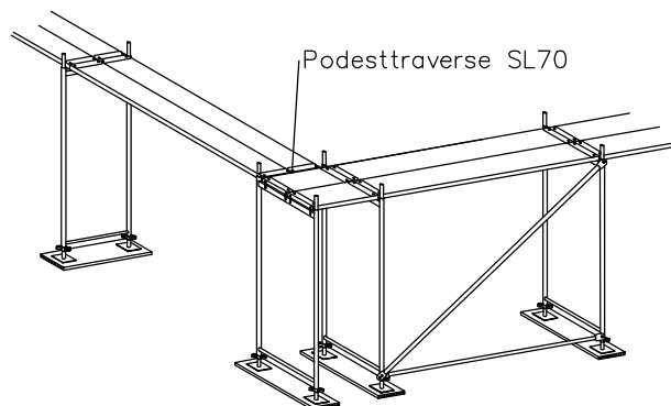
Bild 7: Eckausbildung (Variante 2)
