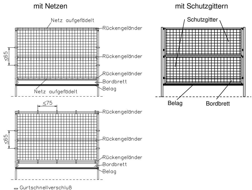
Bild 28: Schutzwand
