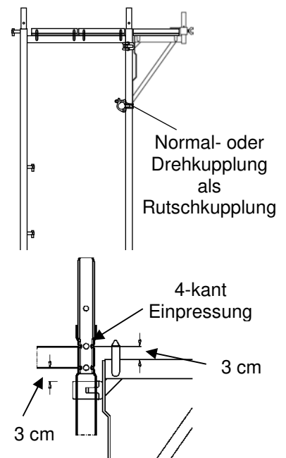
Bild 24: Konsole 64
