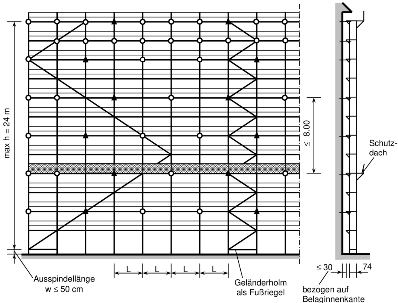
Bild 33: Konsolvariante 2 (Konsole 74 ohne lange Strebe), L = 3.00 m ohne Schutzwand in der obersten Ebene, Ankerraster: 8 m versetzt unbekleidet vor geschlossener Fassade
