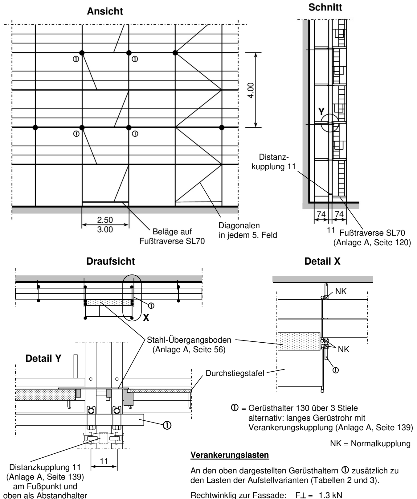
Bild 59: Leitergang
