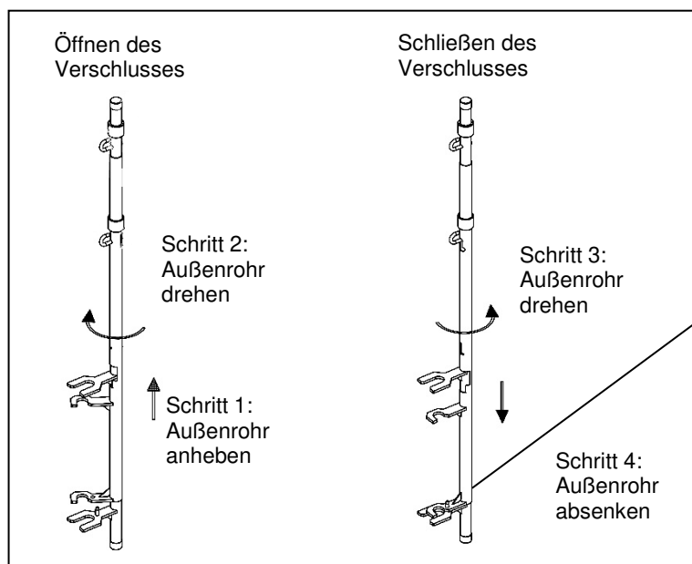
Bild 9: Funktionen des MSG-Pfostens
