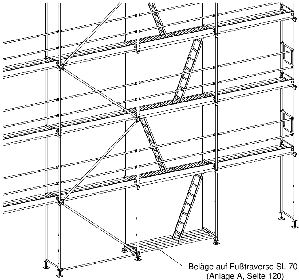
Bild 16: Innen liegender Leitgang
