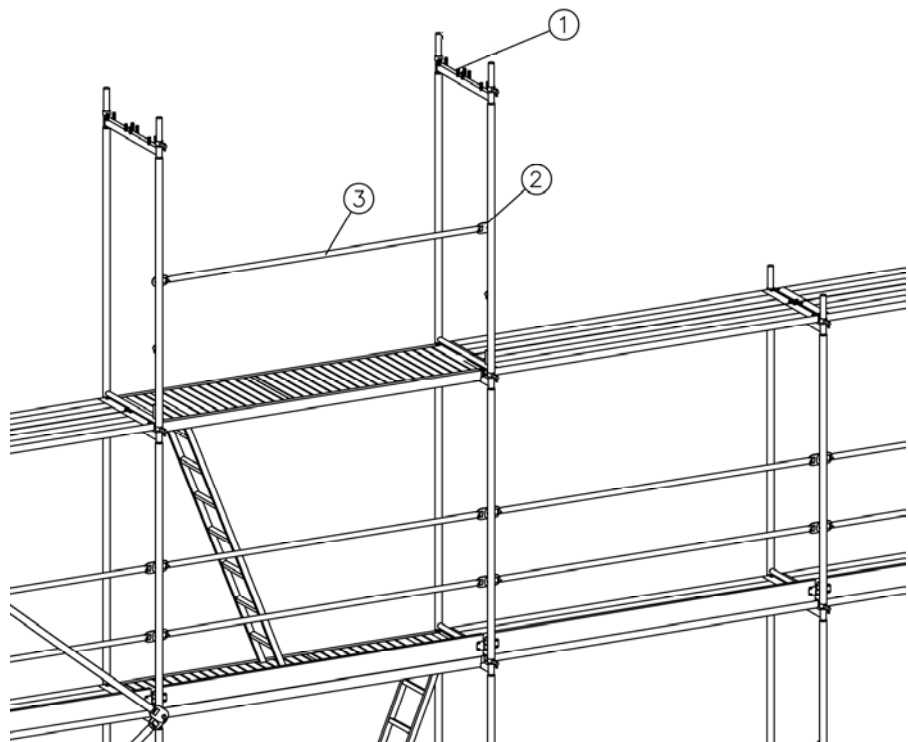
Bild 13: Geprüfte Anschlagpunkte
