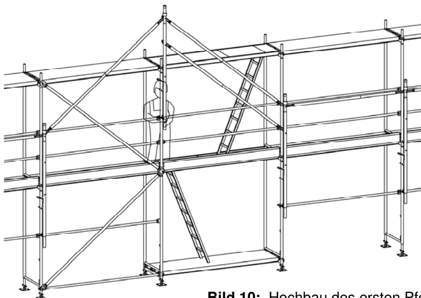
Bild 10: Hochbau des ersten Pfostens
