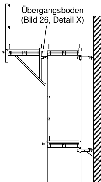
Ausführung mit 1 Kupplung
